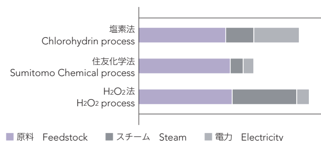
各製法のエネルギー原単位比較 (kcal/kg-PO)
